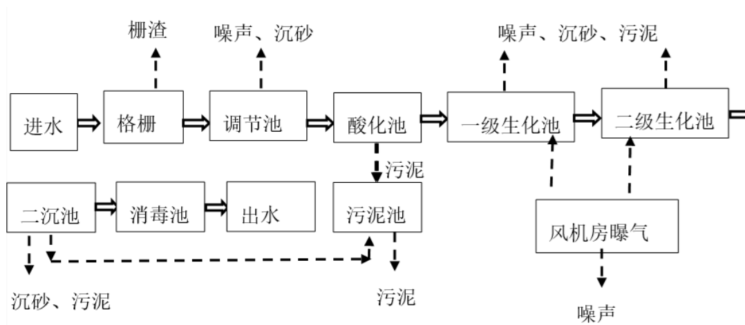
图 3.10-7 车河镇污水处理站生化处理工艺流程图
