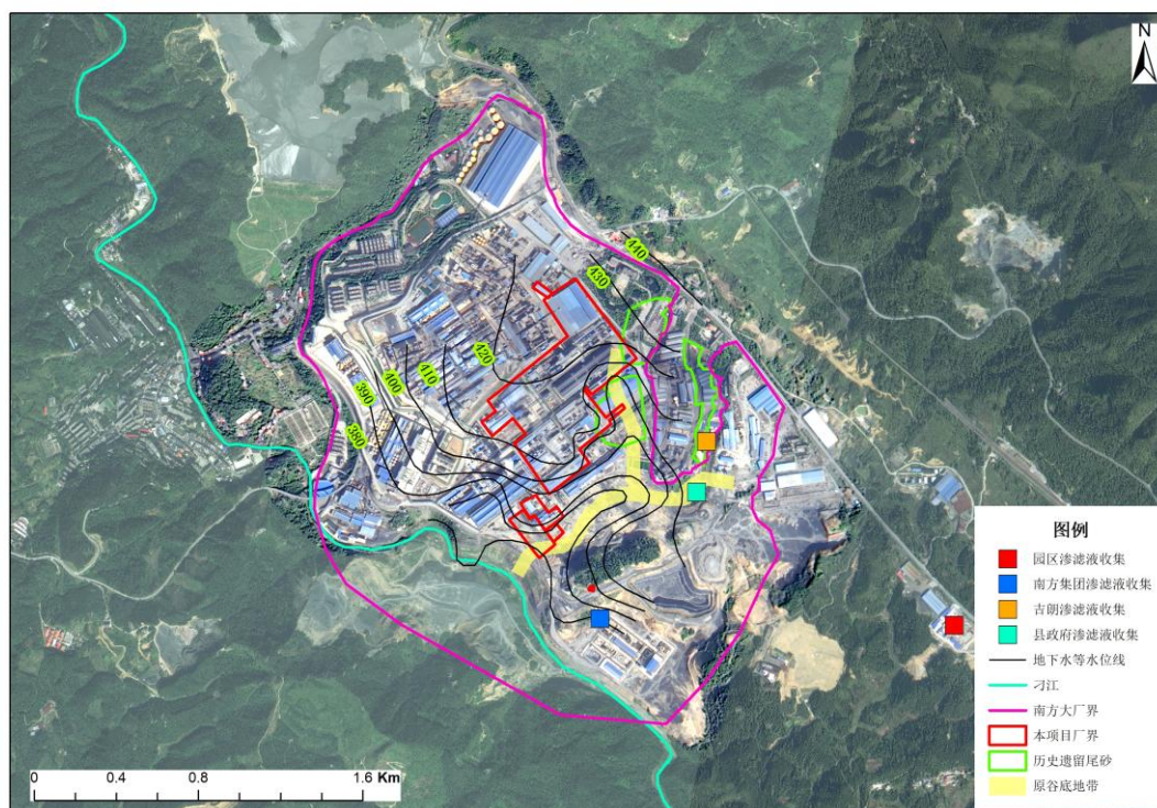
图 4.9-1 渗滤液收集措施位置示意图
