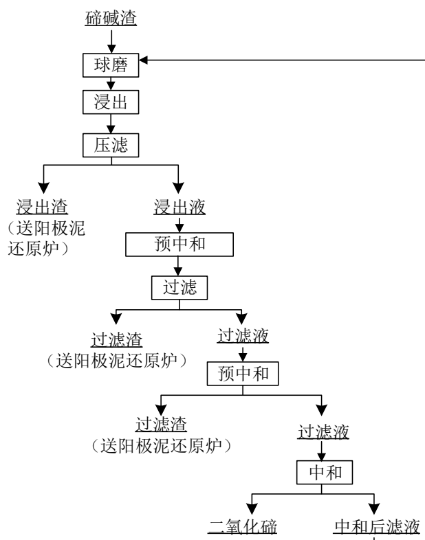
图 3.3-3 二氧化碲生产工艺流程图
