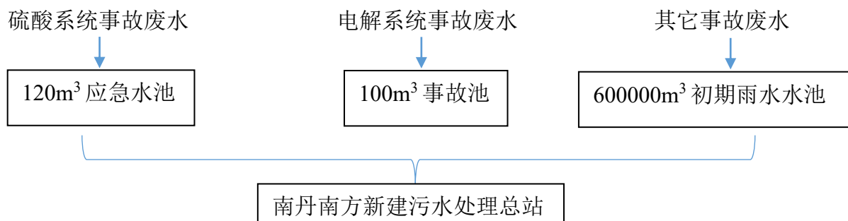
图 3.8-1 改扩建项目事故污染控制图
